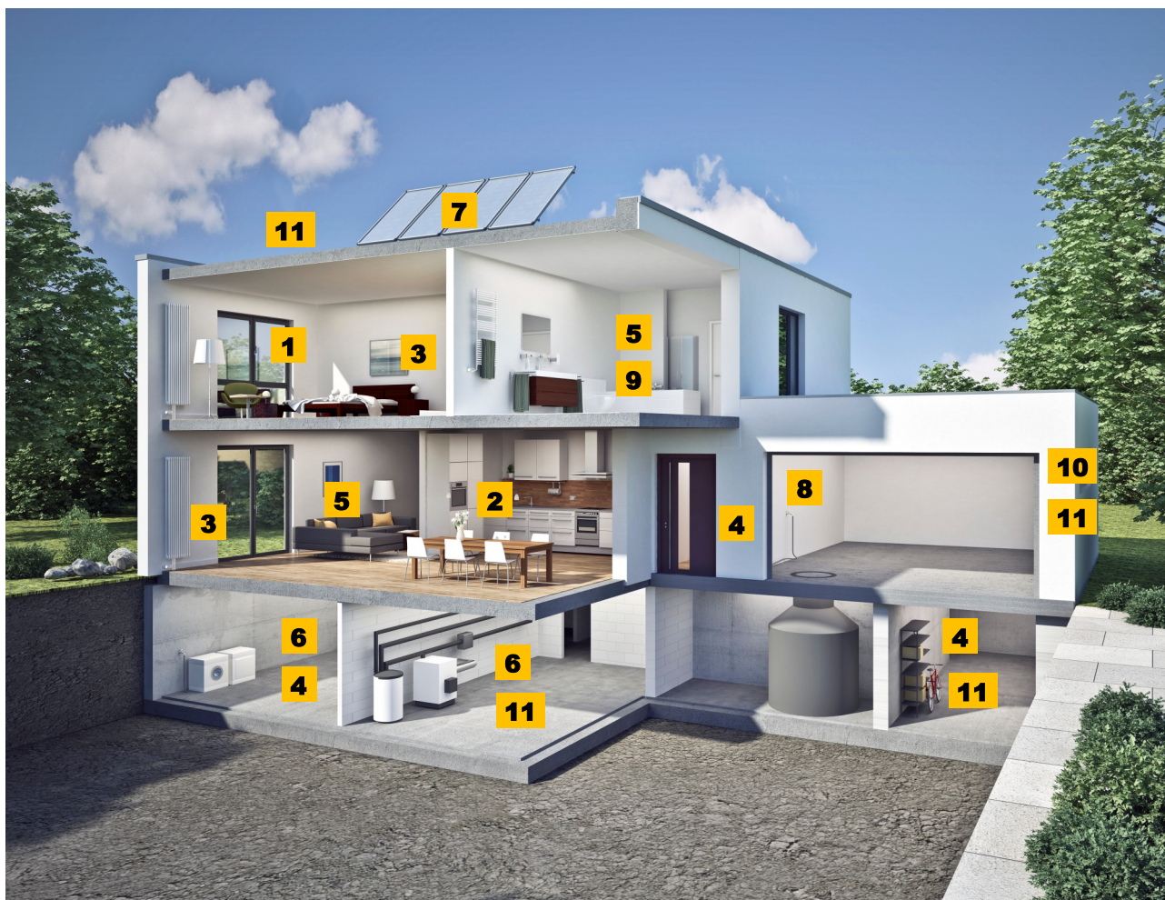
Abbildung: Veranschaulichung möglicher Systeme und Funktionen in einem heutigen Smart Home Standard, inkl. deren Erklärung auf der Folgeseite.
